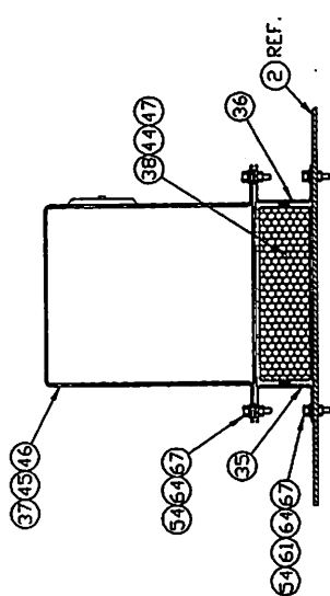
SECTION D-D SCALE: 2=1
